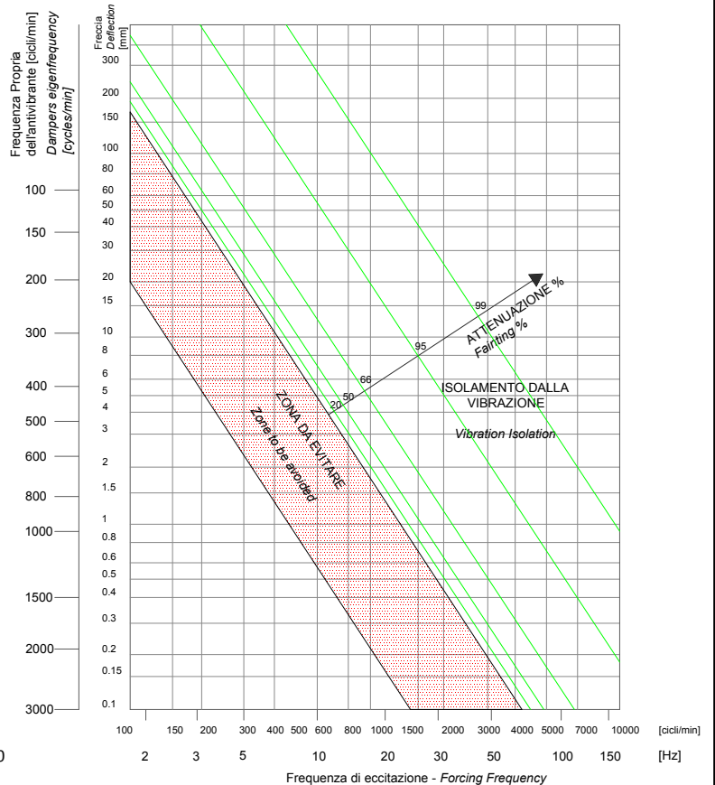
GRAFICO DELL'ISOLAMENTO - Isolation diagram
